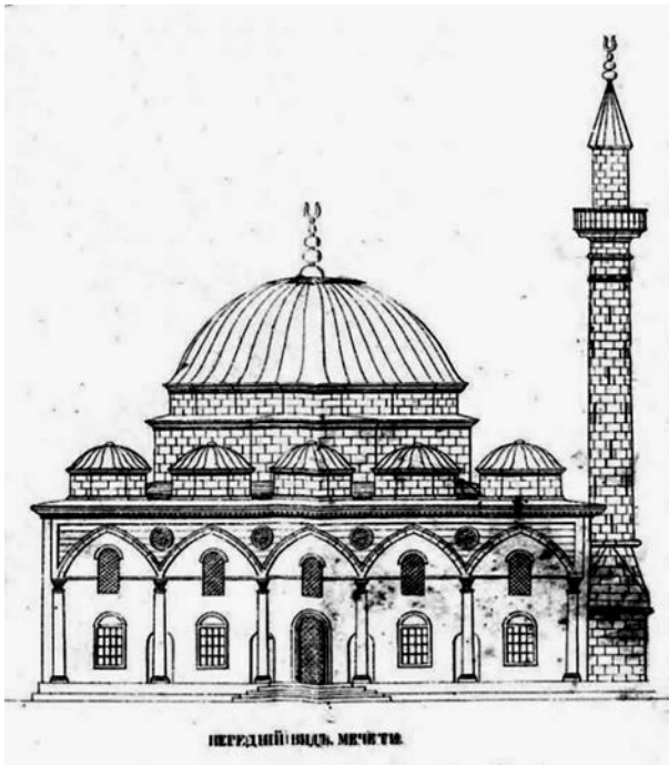
Рис. 7. Загальний вигляд мечеті Сулеймана (Біюк-Джамі) в Кефе з півночі. Креслення XIX ст.
